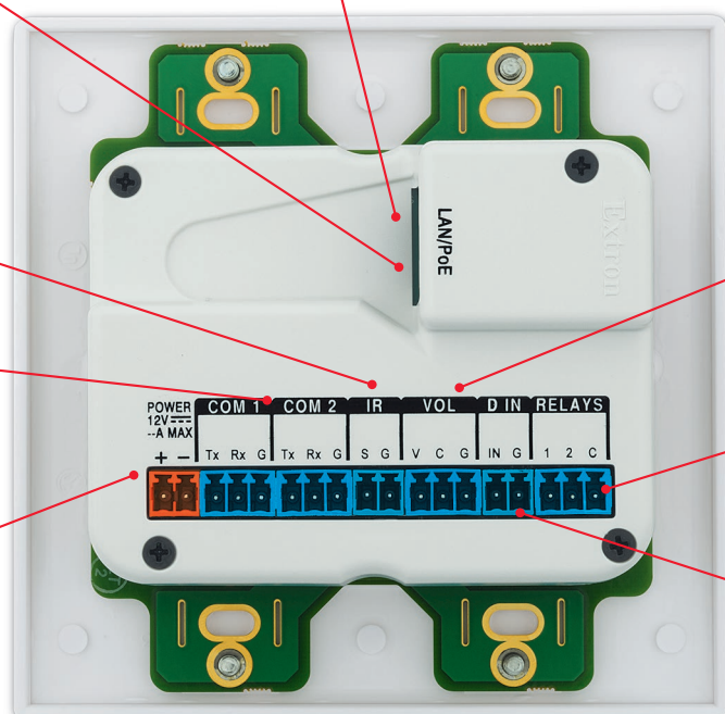
MLC Plus 84 D - Panneau arrière
